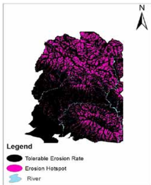
नक्सा: लोथर-पम्फा जलाधार भित्र भू-क्षयको अवस्था
